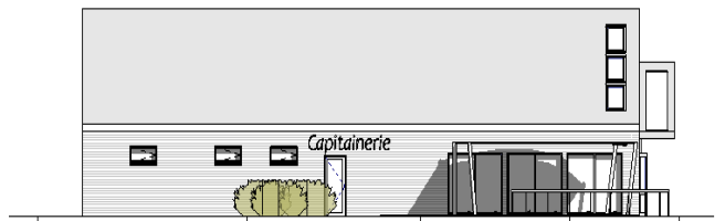
Façades Sud et Est 1/100e
