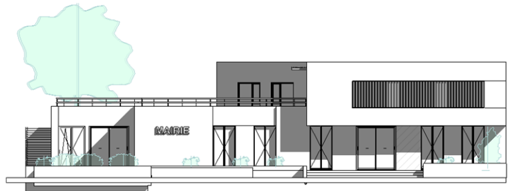
Façade Sud Est- échelle 1/200
