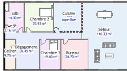
Plan RdC
