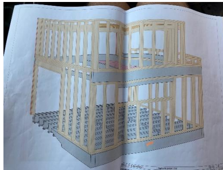
Chantier extensions OB 25m2 isolation laine de bois à Lyon – Façades viroc
