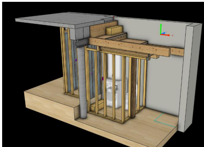
Partie d'une maison escalier et toilette - Projet perso
