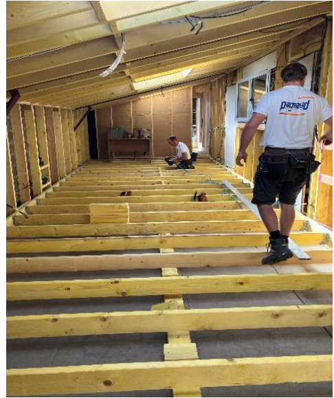
Extension des bureaux de l'entreprise en OB à Nantes
